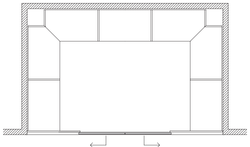
Struttura armadio angolare a "C" prof. cm. 58 con 2 fianchi in profondità superiore. 2 porte scorrevoli complete di binario
