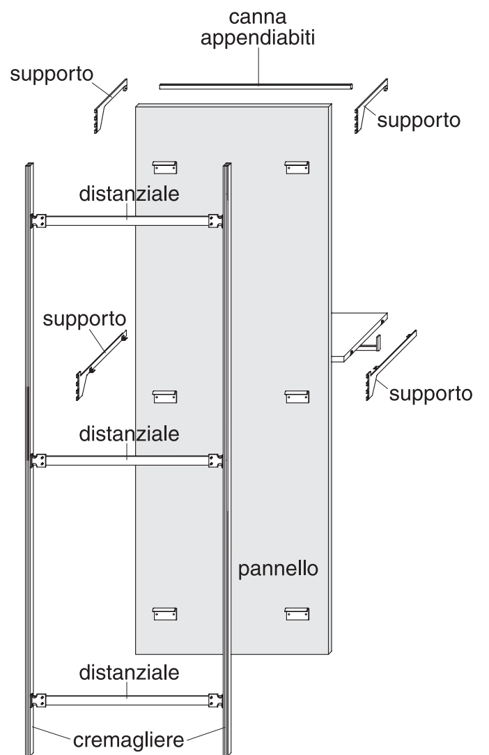
VISTA POSTERIORE
