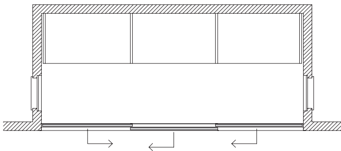
Struttura armadio prof. cm. 58 3 porte scorrevoli complete di binario
