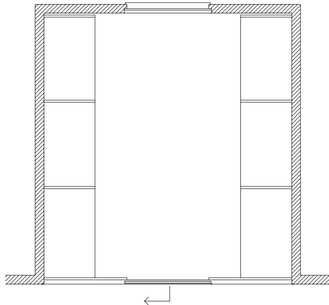
Strutture armadio prof. cm. 58 con 2 fianchi in profondità superiore. 1 porta scorrevole completa di binario.
