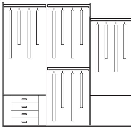
Binari superiori L. cm. 301 con 3 tagli fuori squadra
