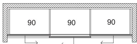
Struttura armadio da muro a muro con fianchi prof. cm. 58
