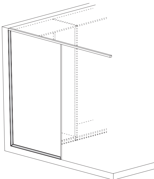
CON PROFILI IN ALLUMINIO
