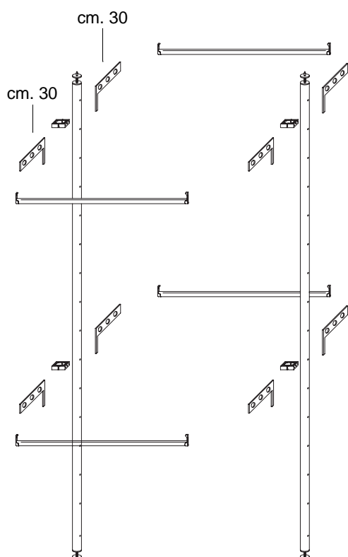
4 staffe con 2 canne appendiabiti fino a L. 93 (occorrono 2 ganasce)
