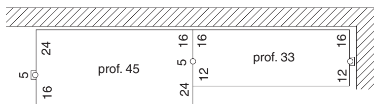
CAMBIO DI PROFONDITÀ ANTERIORE
