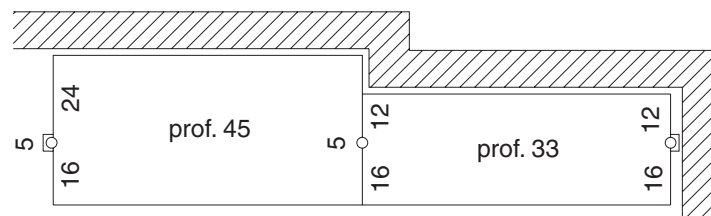
CAMBIO DI PROFONDITÀ POSTERIORE
