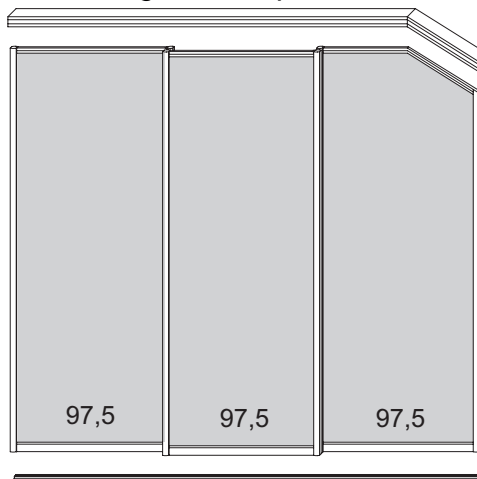
Binario inferiore L. cm. 286
