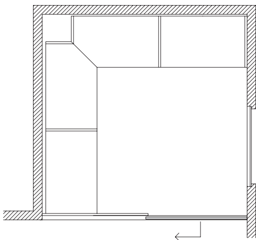
Struttura armadio angolare a "L" prof. cm. 58 con 1 fianco in profondità superiore. 1 porta scorrevole completa di binario.
