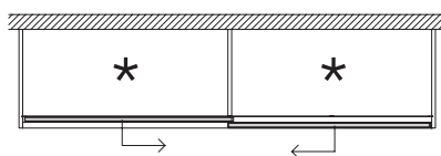
2 porte scorrevoli (per armadio superiore a L. 250 considerare porte MAXI FLOOR)
